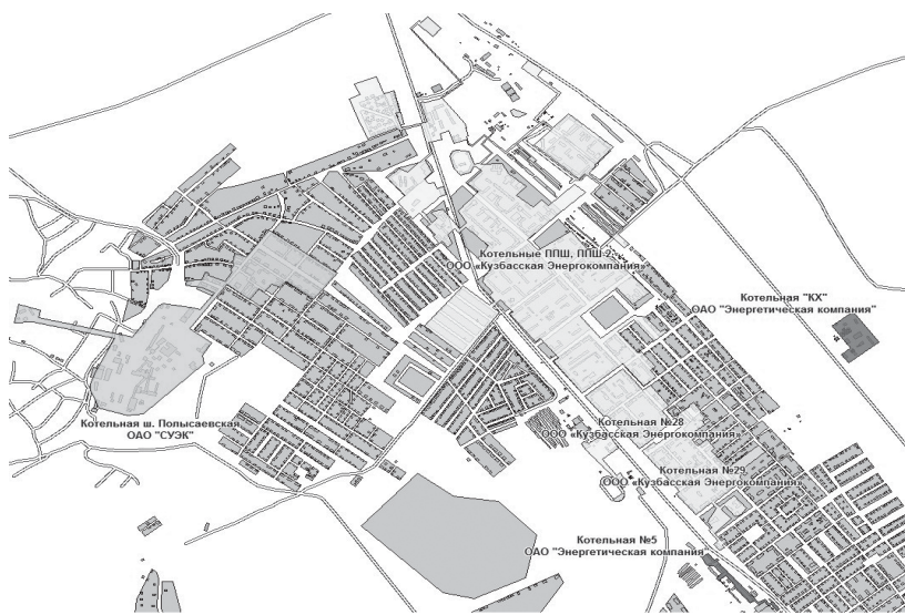
Рис. 2.3. Перспективные зоны действия источников теплоты в системе теплоснабжения Полысаевского городского округа по состоянию на 2030 г.
